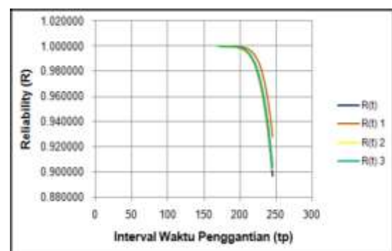
Gambar 5.2 Grafik Perbandingan Nilai R(t) Komponen Modulator jika Parameter \beta , Y , \eta Dinaikkan
