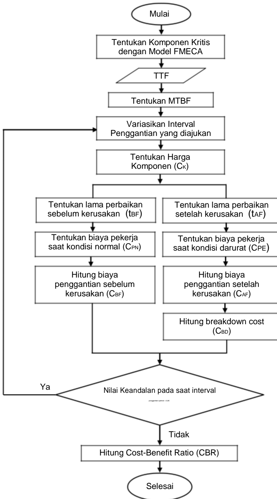
Gambar 3.1 Diagram Alir Model Penentuan Interval Waktu Penggantian Komponen Kritis III-7
