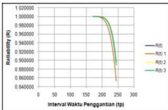
Gambar 5.2 Grafik Perbandingan Nilai R(t) Komponen Modulator jika Parameter \beta , Y , \eta Diturunkan
