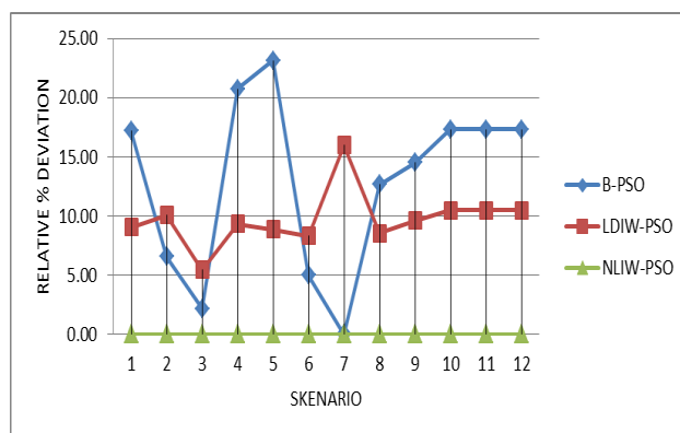
Gambar 11. Grafik performansi algoritma
