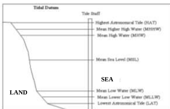
Fig.5 Tidal datum
